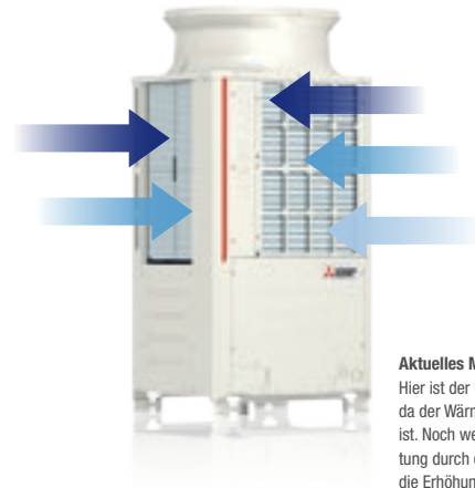
Altes Modell (YLM) In Bereichen, die weiter vom Lüfter entfernt sind, wird der Luftdurchsatz wegen des dreiseitigen Luftansaugsystems und des vertikal positionierten langen Wärmetauschers vermindert.
