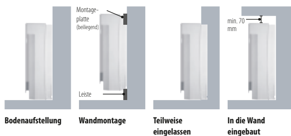
Flexible Montage mit 4 Einbaumöglichkeiten
